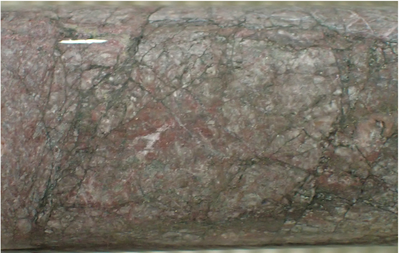
Abb. 2: Bruchbrekzien und Pyrit verwitterter Senit am Anfang des Bohrlochs DO-19-255
