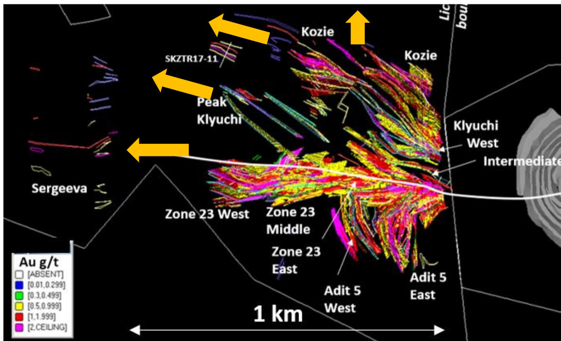
Abbildung 1. Draufsicht des Blockmodells für die erste Mineralressource bei Sergeevskoe und Explorationsziele in den westlichen und nordwestlichen Erweiterungen. Die mineralisierten Abschnitte in den historischen Löchern sind in grau-blauer Farbe dargestellt.
