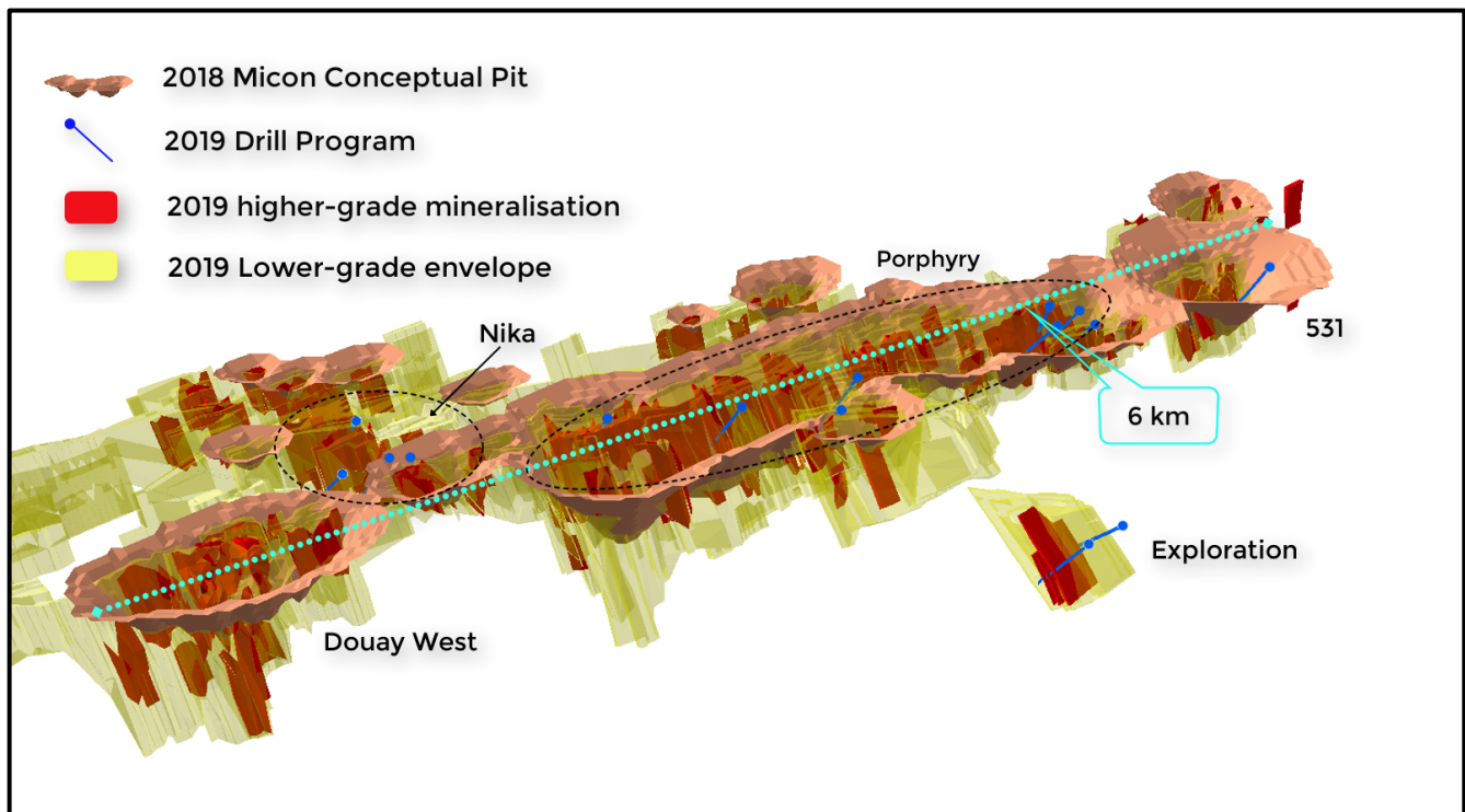
Abb. 1: 3D-Mineralisierungsmodell von Maple Gold mit konzeptionellen Gruben und Verteilung der Bohrungen aus dem Winter 2019-Programm.
