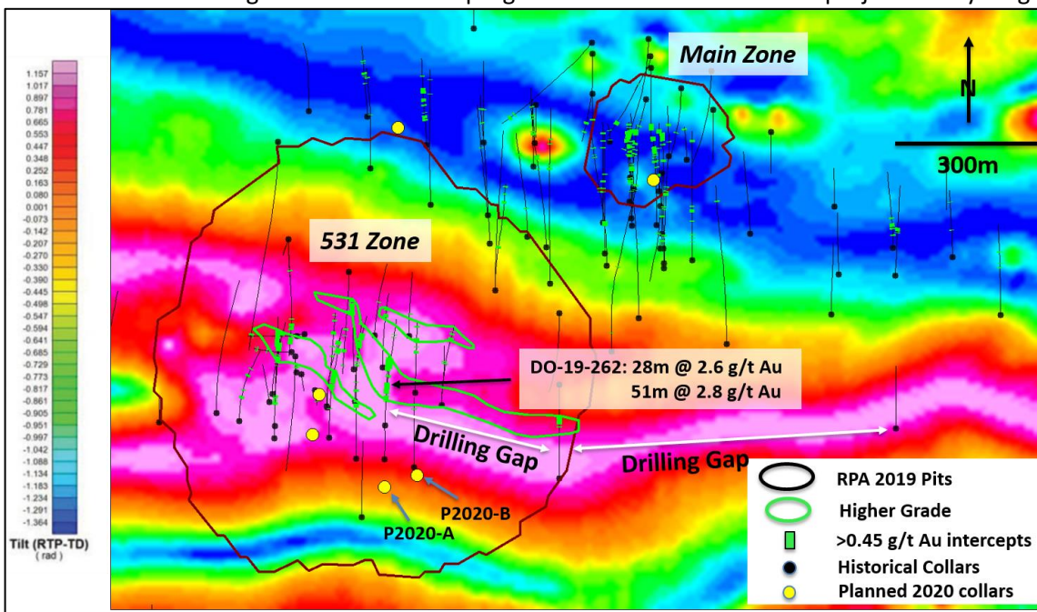
Abb. 2: Bohrplan für den gesamten Bereich der 531 Zone mit bei reduzierter Polneigung abgeleiteter Magnetik (RTP-TD) zur Hervorhebung lithologischer Kontakte. Beachten Sie die große Bohrlücke unmittelbar ost-südöstlich und östlich der höhergradigen Abschnitte in DO19-262. P2020-A wird zurzeit niedergebracht. Zusätzlich zu den geplanten Step-Out-Bohrungen und Bohrungen in den Lücken innerhalb des bekannten Ressourcenbereichs plant das Unternehmen auch, einen Teil seiner Explorationsbudgets für 2020 für neue Goldentdeckungen an anderer Stelle auf der Liegenschaft zur Verfügung zu stellen. Das Unternehmen wird in
