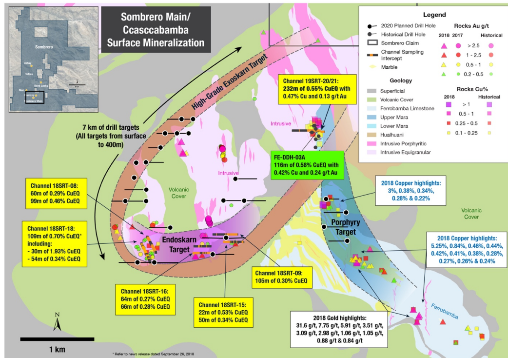
Abbildung 1: Veranschaulicht den vorgeschlagenen Bohrplan auf dem Sombbrero-Hauptzielgebiet. Die DIA ermöglicht es Auryn, bis zu 33 Löcher von 23 Plattformen aus zu bohren.
