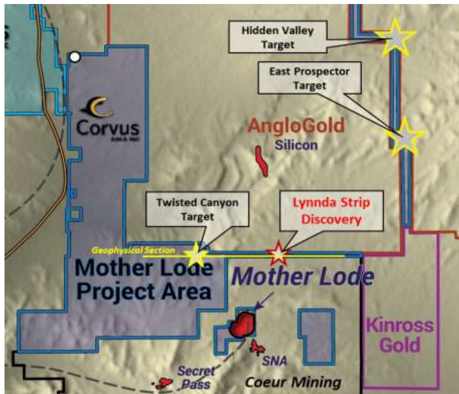
Abb. 1: Standort von Lynnda Strip und anderen Zielen im Mother Lode Belt (Nevada)
