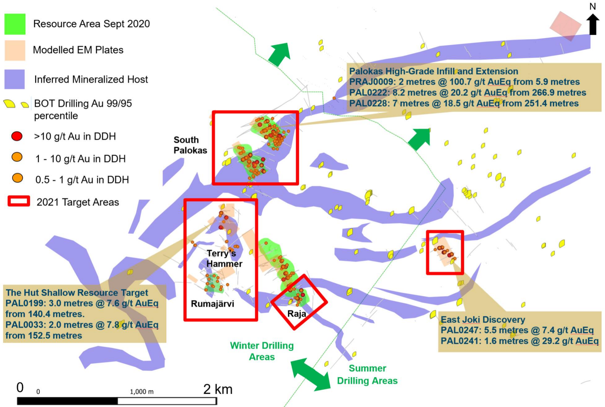
Abbildung 1: Das Projekt Rajapalot in Finnland mit den EM-Platten, dem abgeleiteten stratabunden Wirt, den Ressourcengebieten und den wichtigsten Zielgebieten für das Bohrprogramm zur Ressourcenerweiterung 2021.
