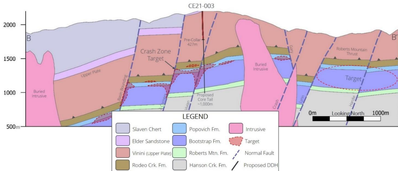
Abbildung 2: Schematischer Profilschnitt B-B', der die Bohrung CE21-003 zeigt, die auf die Wirtsgesteine der Lower Plate der Popovich- und Bootstrap-Formation im Liegenden der Verwerfungszone Four-Corners abzielt.
