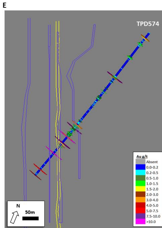
Abbildung 8: Hochgradiges Bohrprogramm Querschnitt, NW-Bereich (E-E')
