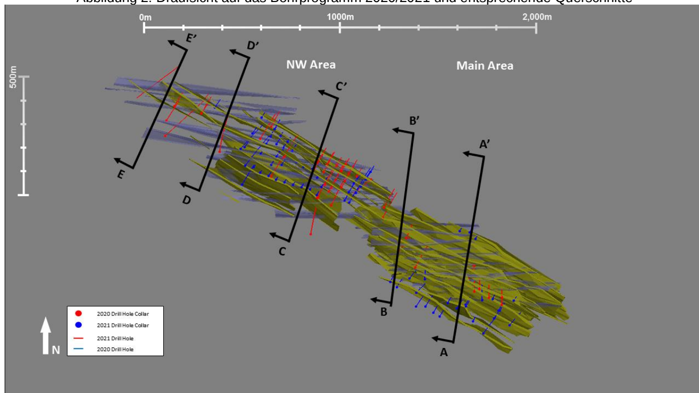
Abbildung 2: Draufsicht auf das Bohrprogramm 2020/2021 und entsprechende Querschnitte
