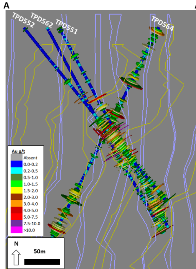
Abbildung 4: Querschnitt des hochgradigen Bohrprogramms, Hauptgebiet (A-A')
