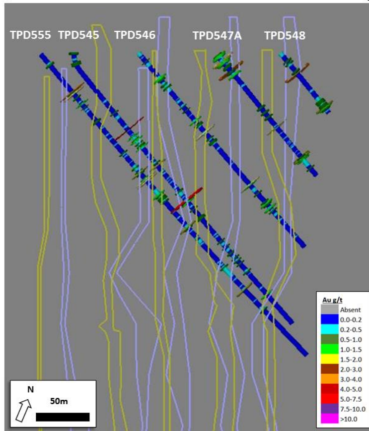
Abbildung 6: Querschnitt des hochgradigen Bohrprogramms, NW-Bereich (C-C')
