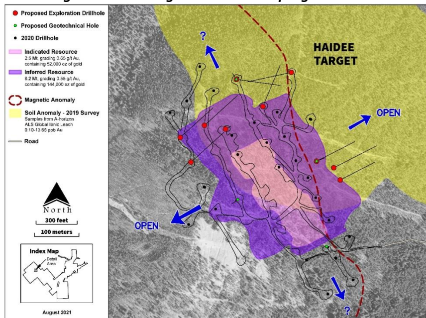
Abbildung 2: Haidee-Zielgebiet 2021 Bohrprogramm
