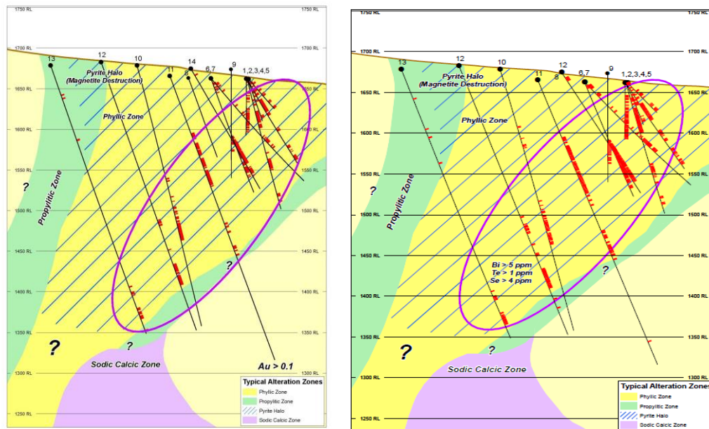
Abbildung 2 – Querschnitt von San Javier mit Abschnitten mit einem Gehalt von >0,1 g/t Au (links) und Bi-/Te-/Se-Anomalien (rechts)
