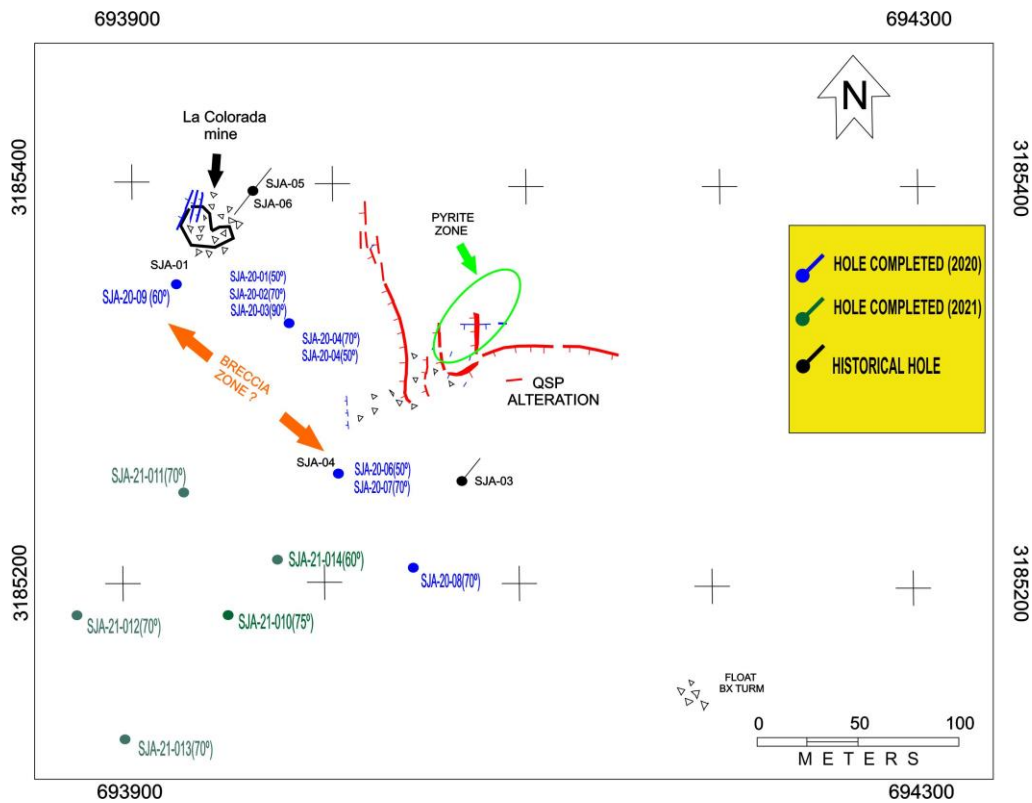
Abbildung 1 – Lageplan der Bohrlöcher bei San Javier
