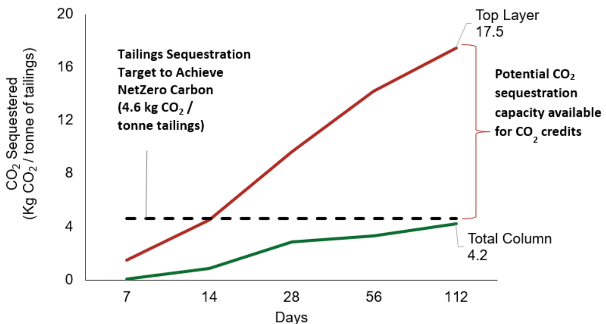
Abbildung 2. Kohlenstoff-Sequestrierungspotenzial von Crawford Tailings
