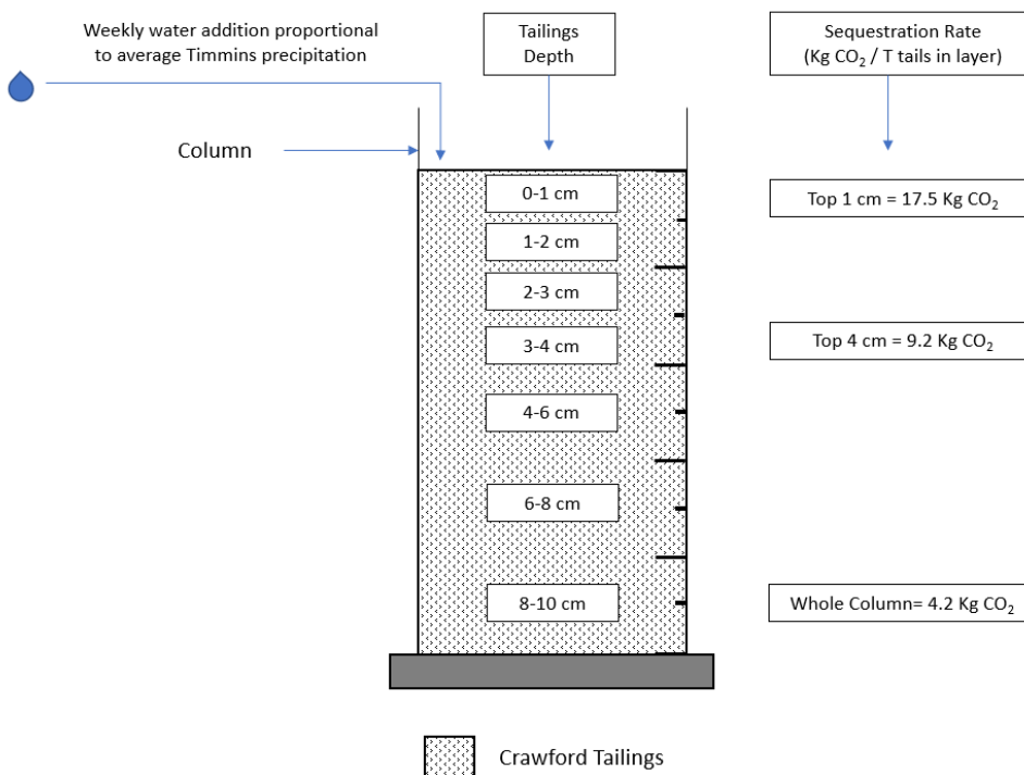
Abbildung 3. Kohlenstoffabscheidungsrate in Abhängigkeit von der Tiefe in Säulenzelltests nach 112 Tagen
