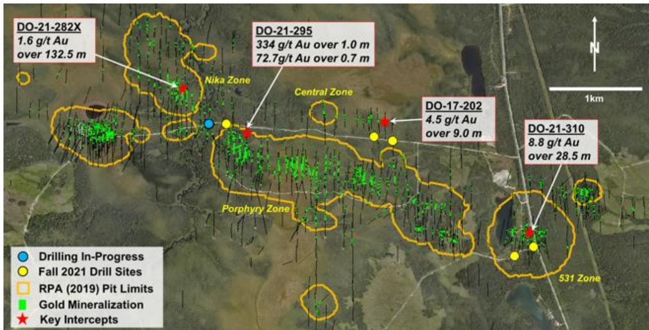
Abbildung 1: Bohrplätze im Herbst 2021. Es sind sechs Bohrungen geplant, um diese zu erproben: 1) die nur spärlich bebohrte Lücke zwischen den Zonen Nika und Porphyry; 2) die östliche Kontinuität der Goldmineralisierung in der Zone Central; und 3) die Kontinuität des besten bisher gebohrten Abschnitts in der Zone 531 nach oben und unten.
