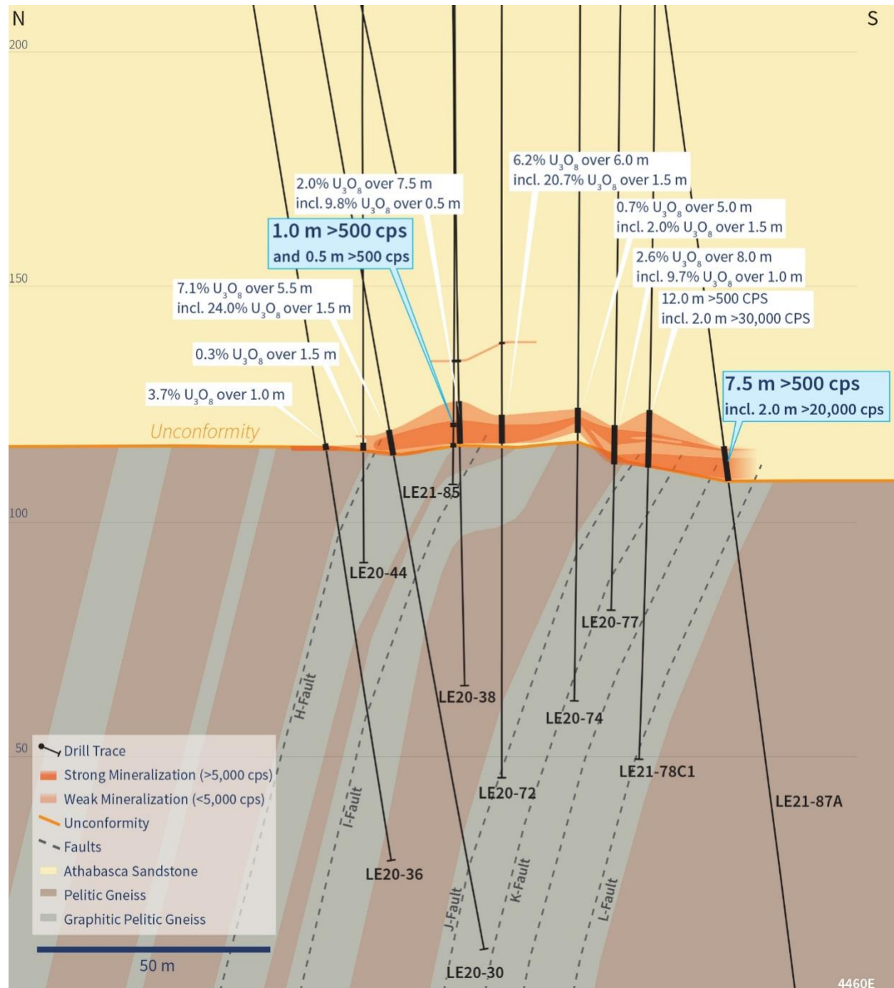
Abbildung 4 - Abschnitt 4460E
