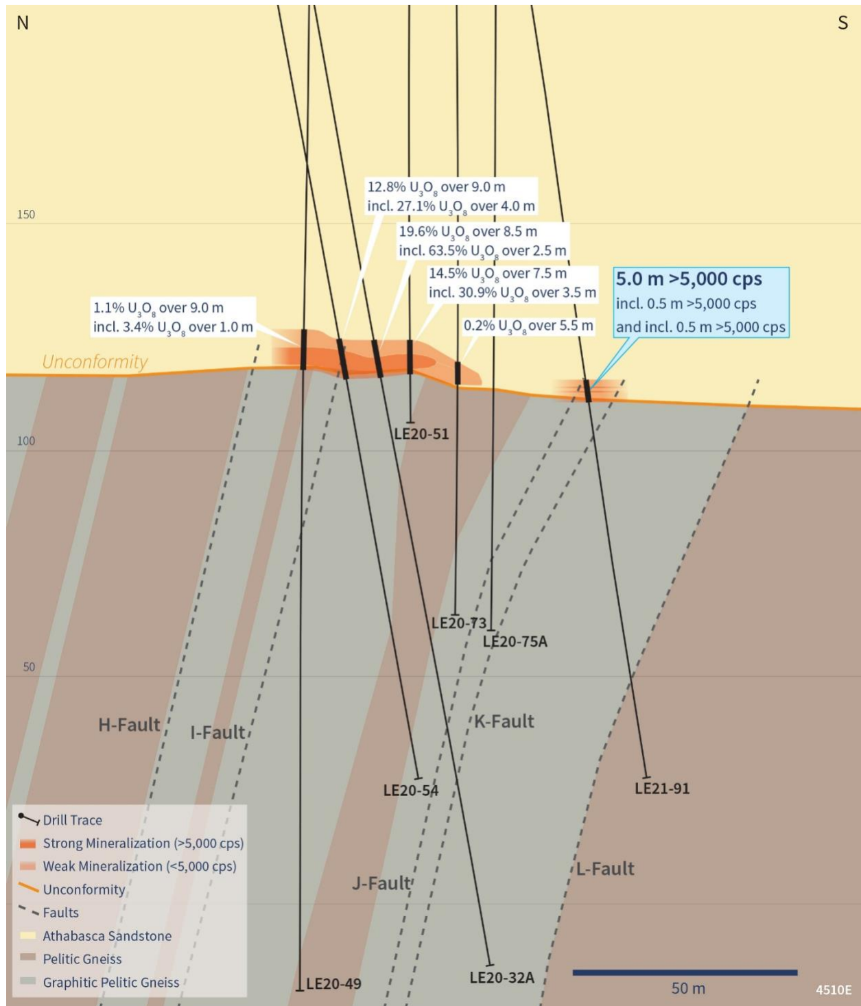
Abbildung 5 - Abschnitt 4510E
