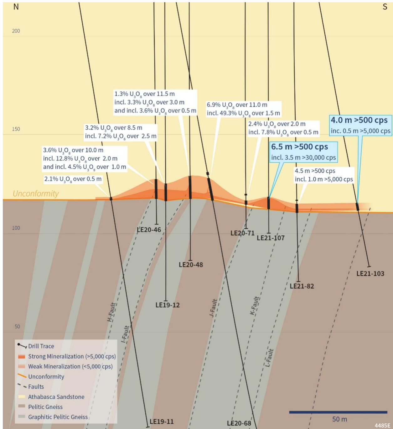
Abbildung 3 - Abschnitt 4485E
