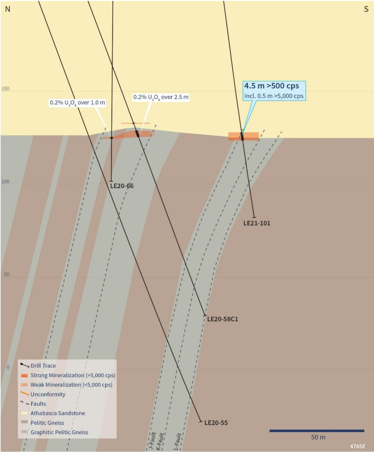
Abbildung 6 - Abschnitt 4785E
