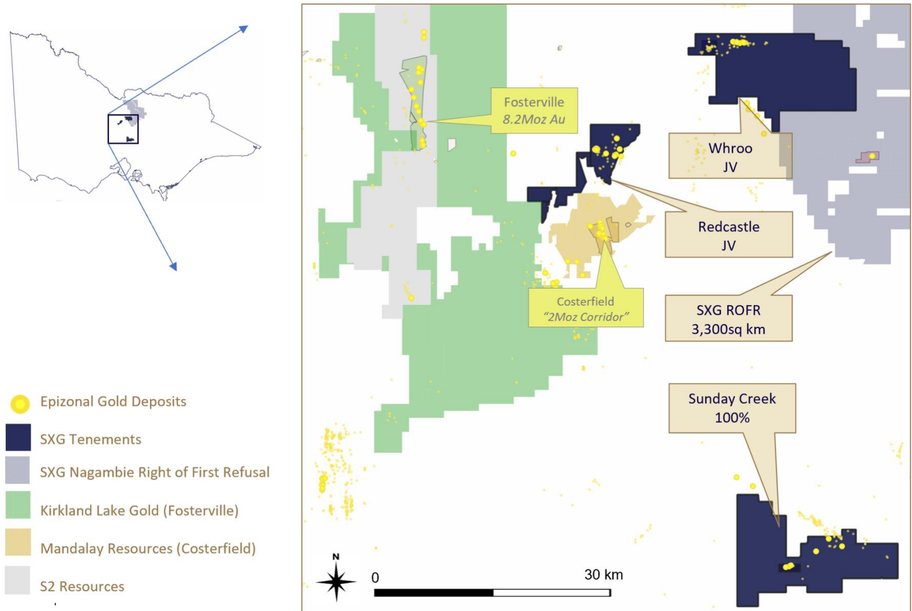
Abbildung 1: Lage der Southern Cross Tenements in Victoria, Australien, mit Schwerpunkt auf 3 der 9 historischen epizonalen Goldlagerstätten
