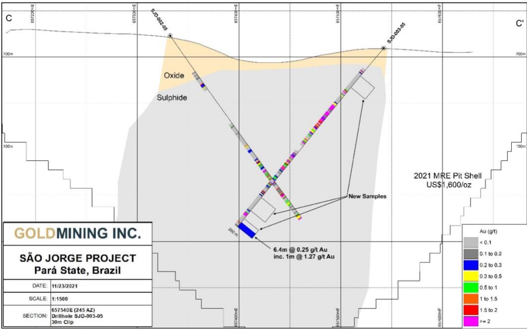
Abbildung 4 - Der nach Nordwesten ausgerichtete Abschnitt 657540E zeigt die Probennahmeergebnisse des Bohrlochs SJD-003-05 aus dem Abschnitt 244-250,4 m.
