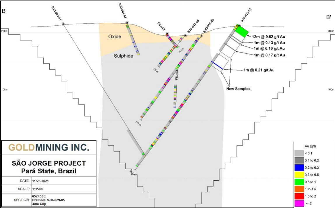
Abbildung 3 - Der nach Westen ausgerichtete Abschnitt 657450 zeigt die Ergebnisse der oberflächennahen Probenahme in Bohrloch SJD-029-05, das einen Abschnitt von 0,0 bis 12,0 m mit einem mineralisierten Saprolit enthält. Beachten Sie, dass dieser mineralisierte Abschnitt ebenfalls weit außerhalb der Grenzen der aktuellen modellierten Mineralisierung vorkommt (schattierter Bereich im Abschnitt).
