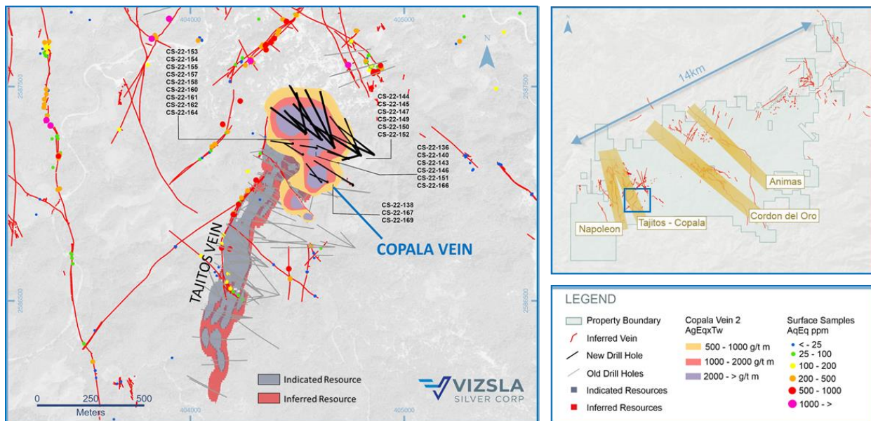
Abbildung 1: Übersichtskarte der jüngsten Bohrungen, die sich auf die Copala-Ader konzentrieren.
