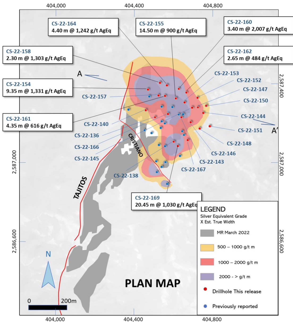
Abbildung 2: Plan der Ader Copala mit Bohrlochdurchstichpunkten.
