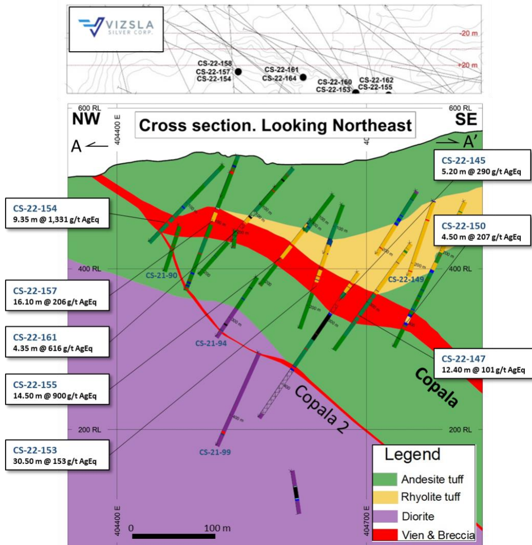
Abbildung 3: Querschnitt durch die Adern Copala und Copala 2.
