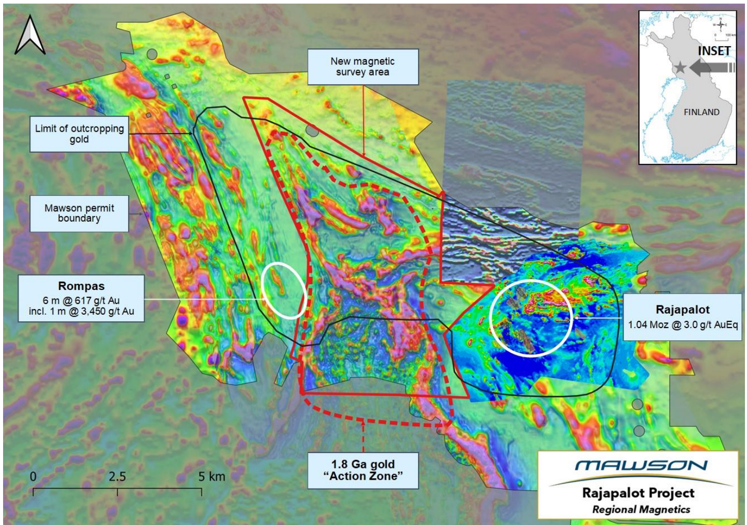
Abbildung 1: Vorhandene magnetische Daten aus Finnland im Zusammenhang mit den Entdeckungen von Rajapalot und Rompas
