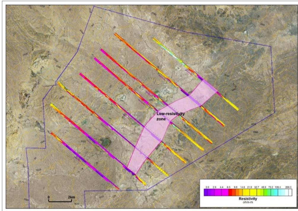
Abbildung 1: Zone mit niedrigem spezifischen Widerstand gegenüber den Abschnitten mit spezifischem Widerstand
