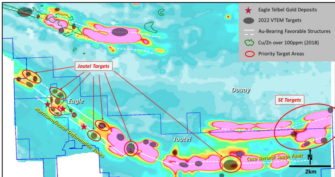
Abbildung 2: Nahaufnahme des Minengebiets Eagle-Telbel und der Liegenschaftsgrenze Douay-Joutel mit identifizierten leitfähigen Zielgebieten und bekannten/interpretierten Strukturen auf einer Tau dB/dt EM-Basiskarte.
