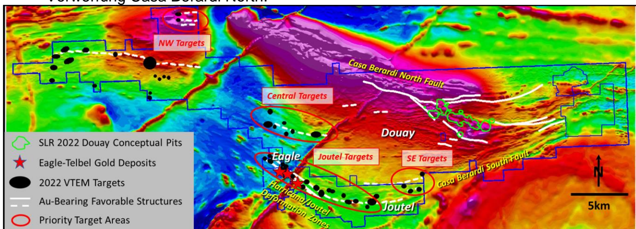
Abbildung 1: Verteilung der leitfähigen Zielgebiete, bekannten goldhaltigen und anderen interpretierten günstigen Strukturen bei Douay (>17 km) und Joutel (>6 km) auf einer residualen magnetischen Basiskarte.
