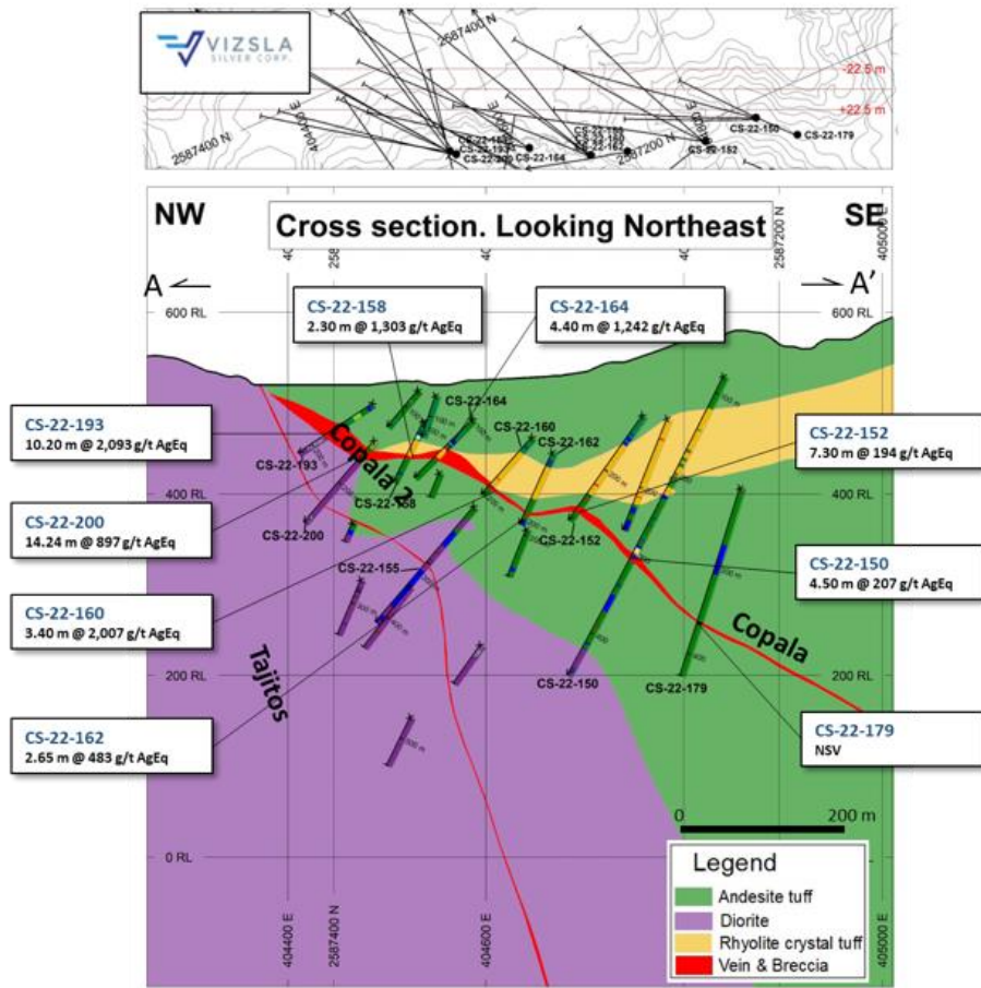
Abbildung 3: Querschnitt durch die Adern Copala, Tajitos und Copala 2.
