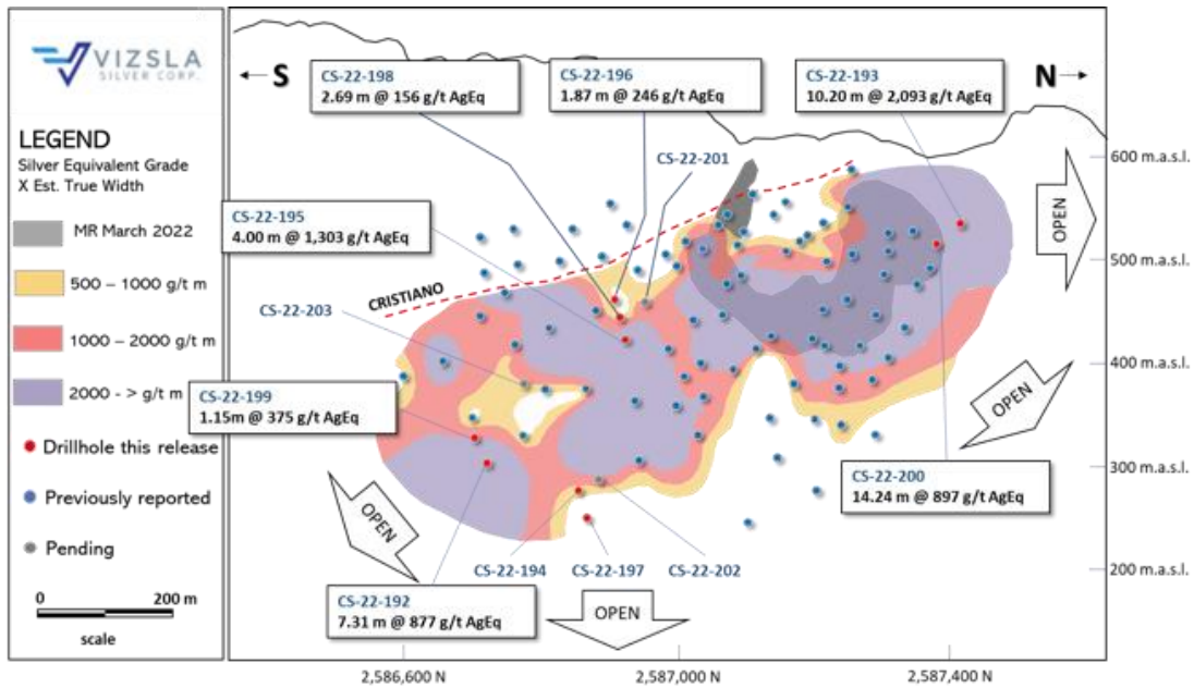
Abbildung 2: Geneigter Längsschnitt für die Copala-Struktur mit Bohrlochdurchstichpunkten. Der Schnitt ist 1x entlang des Streichs und 1,4x entlang der Neigung, um die durchschnittliche Neigung von 46 Grad von Copala auszugleichen.
