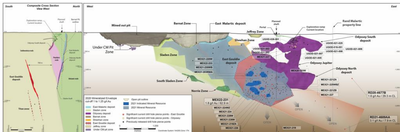
Abbildung 1: Mine Canadian Malartic - zusammengesetzter Längsschnitt
