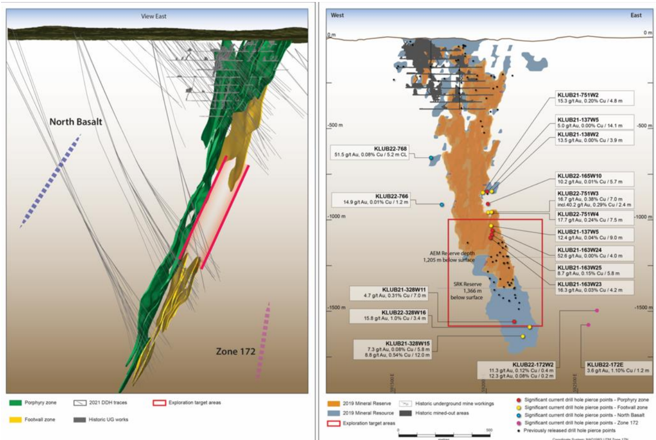
Abbildung 5: Oberer Biber-Verbund-Längsschnitt
