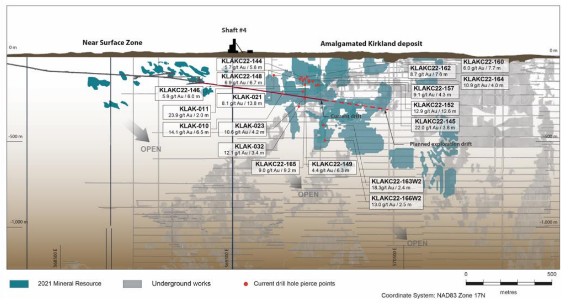
Abbildung 4: AK-Lagerstätte Längsschnitt
