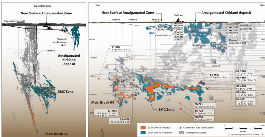
Abbildung 3: Komposit-Längsschnitt der Mine Macassa und der AK-Lagerstätte
