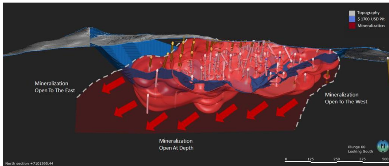
Abbildung 2: Idealisierter Längsschnitt der Rabengrube und MRE-Grenzen
