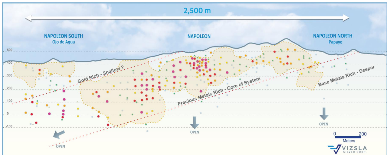
Abbildung 4: Längsschnitt des Explorationsmodells des Erzgangkorridors Napoleon mit Durchstoßpunkten.
