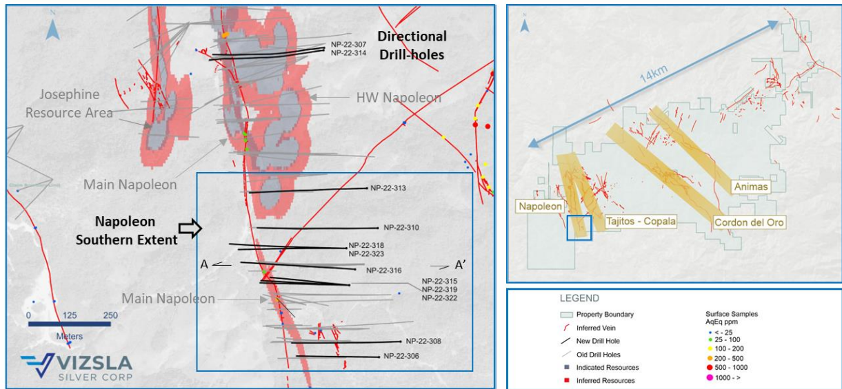
Abbildung 1: Übersichtskarte der jüngsten Bohrungen entlang der südlichen Ausdehnung des Erzganges Napoleon.
