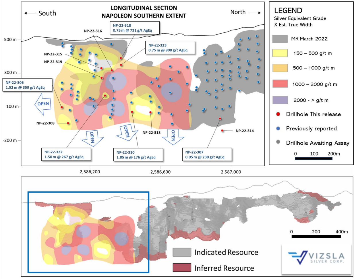
Abbildung 2: Längsschnitt des Haupterzganges Napoleon. Die Sektion ist in Fallrichtung der Struktur geneigt.
