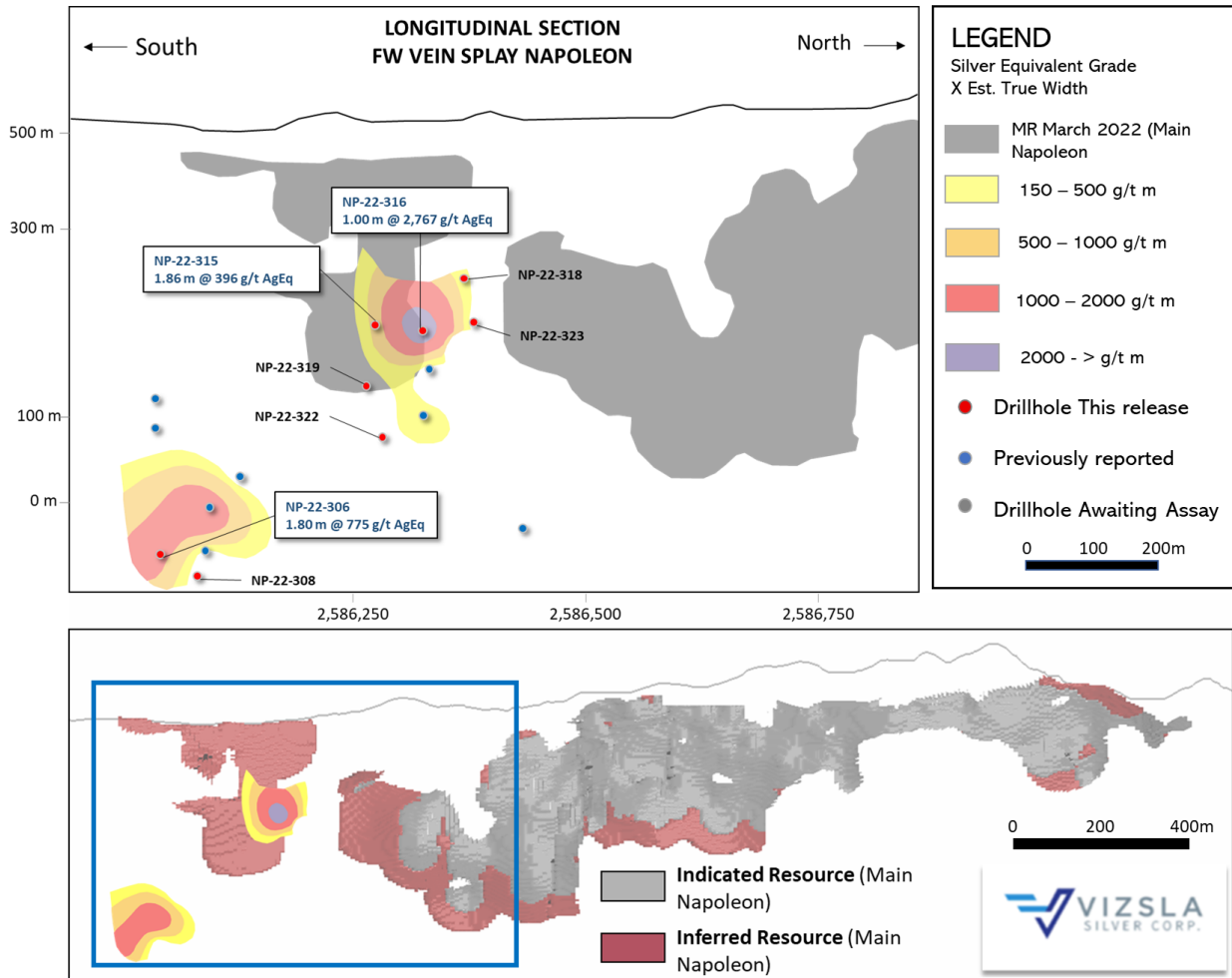
Abbildung 3: Längsschnitt einer Gangverzweigung (FW Splay 1) im Liegenden des Haupterzganges Napoleon. Die Sektion ist in Fallrichtung der Struktur geneigt.
