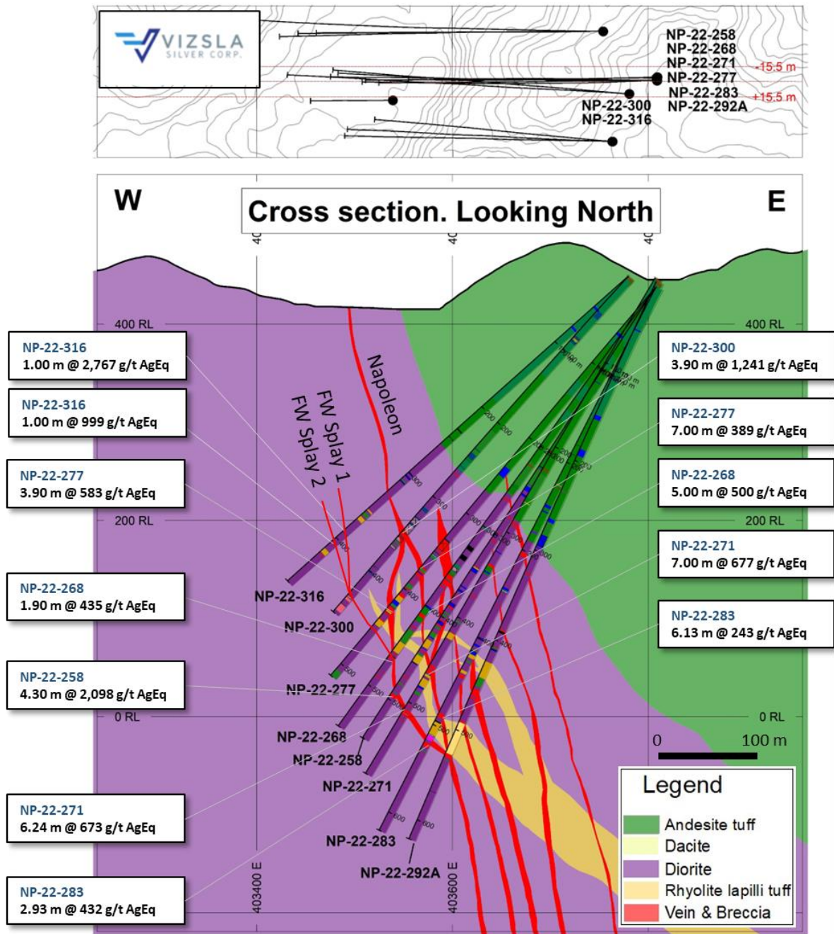
Abbildung 5: Profilschnitt mit Hervorhebung der jüngsten Bohrabschnitte, die sich unterhalb der Grenze der vermuteten Ressource im südlichen Bereich von Napoleon befinden.
