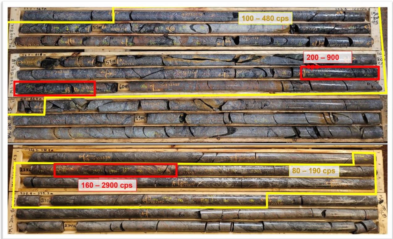
Abbildung 3: Zwei Zonen mit typischer rötlicher Alteration und Uranmineralisierung, die von ML-200 durchteuft wurden.
