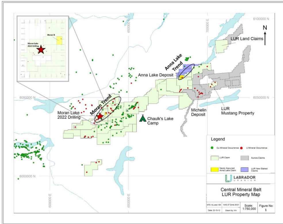
Abbildung 1: Liegenschaften von Labrador Uranium im Central Mineral Belt (Labrador) mit Hervorhebung der Standorte der Bohrungen bei Moran Lake und der Bodenarbeiten im Jahr 2022.
