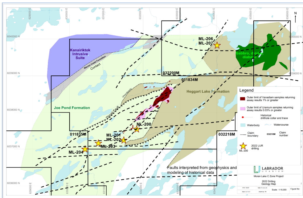
Abbildung 2: Abgeschlossene Bohrungen und aktualisierte Ziele für die Zone Moran Lake C mit unterlagernder Grundgebirgsgeologie. Die Geologie stammt aus dem Bewertungsbericht von Crosshair (Steele, L. und Fox, D., 2012).
