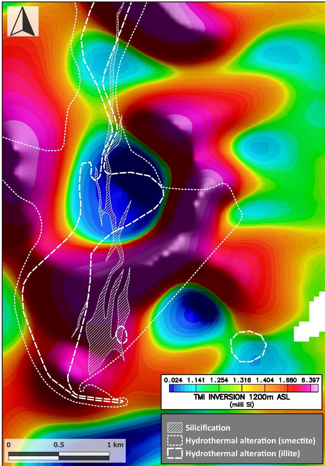
Abbildung 1: Inversionskarte der magnetischen Gesamtintensität auf 1200 m über dem Meeresspiegel (ASL) mit der Verkieselung aus der Kartierung und den hydrothermalen Umwandlungen aus der IR-Spektrometrie (Terraspec) Studie. Illit ist ein Hochtemperatur-Tonmineral, das ein häufiger Bestandteil von
