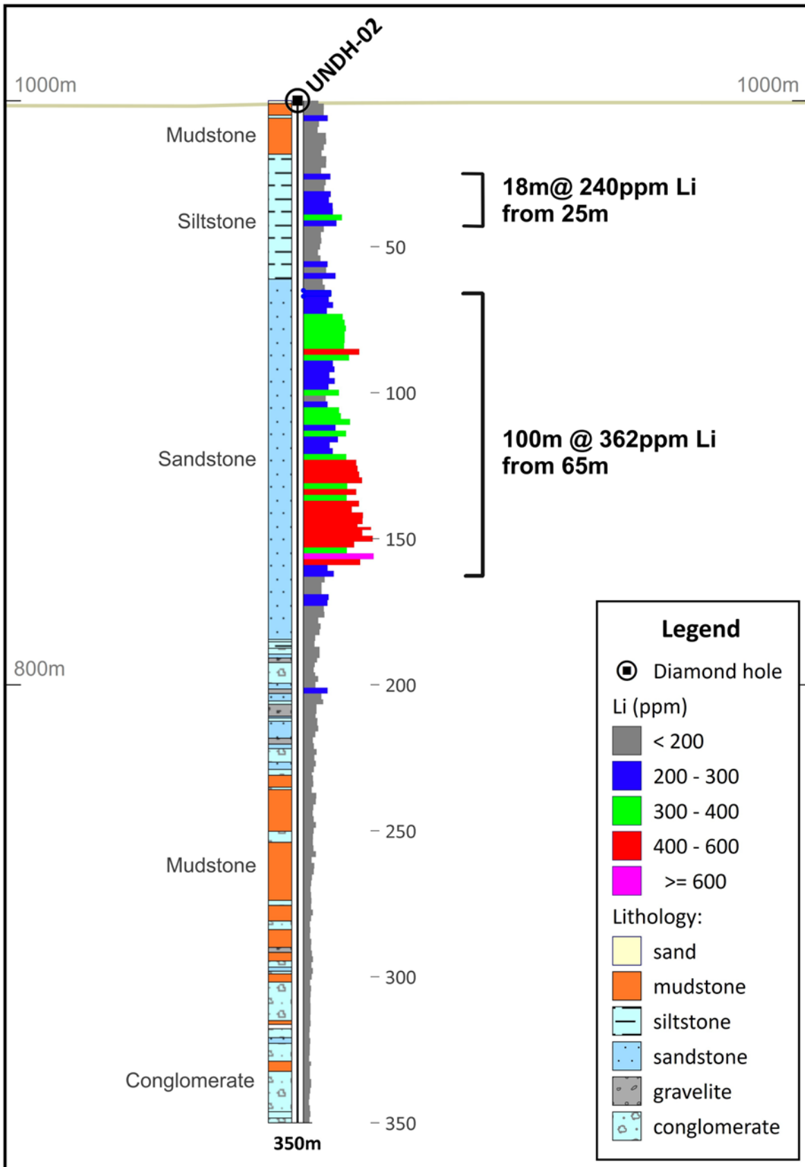
Abb. 3: Lithiumergebnisse von UNDH-02 bei Urgakh Naran in der Mongolei
