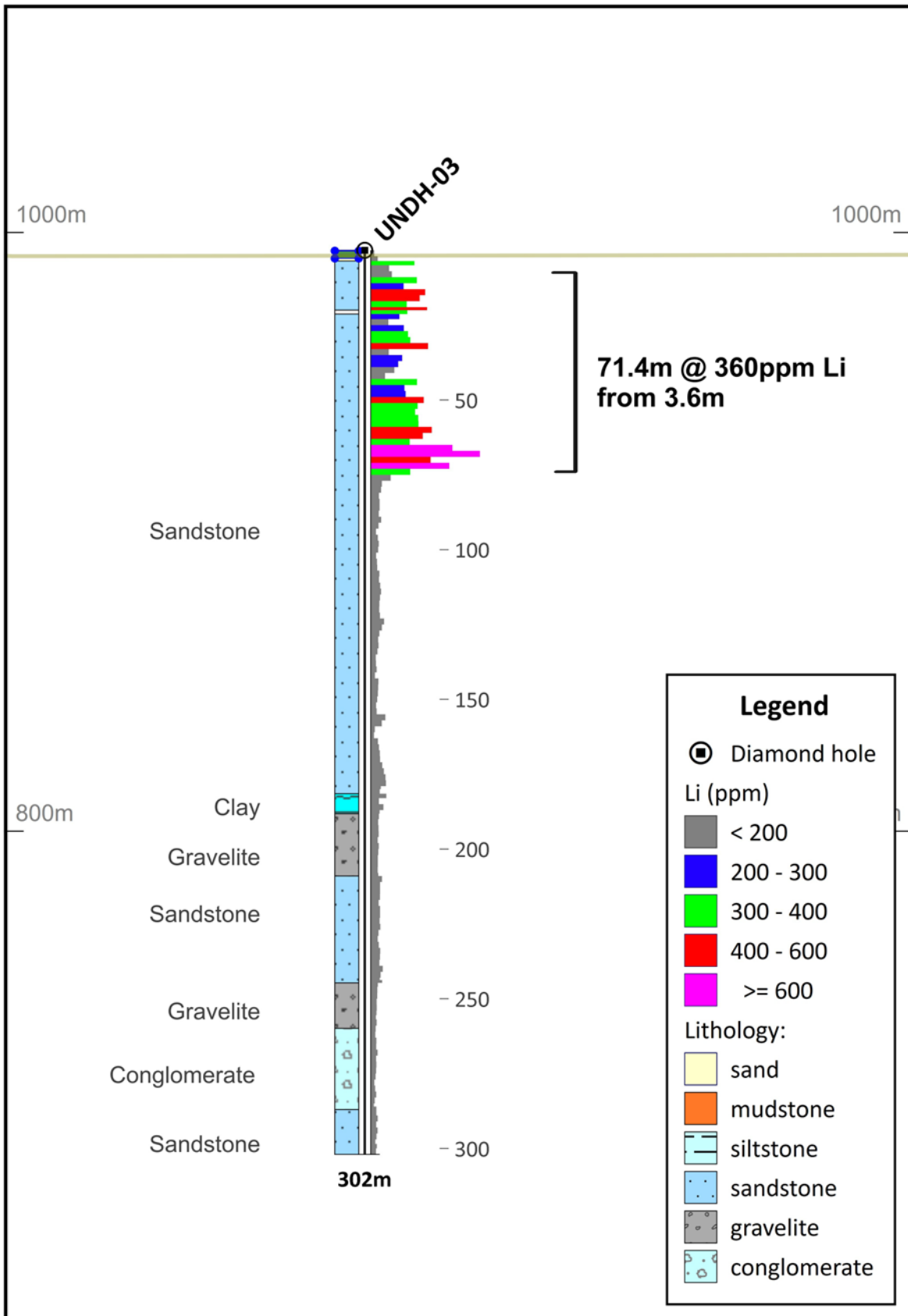
Abb. 4: Lithiumergebnisse von UND H-03 bei Urgakh Naran in der Mongolei
