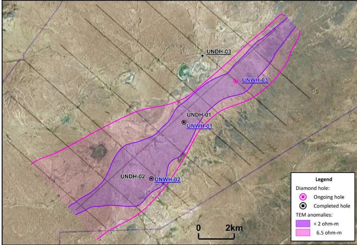
Abb. 1: Karte der Bohrstandorte beim Lithiumprojekt Urgakh Naran in der Mongolei
